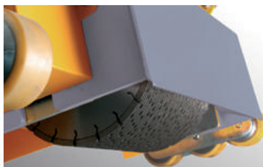
Voll bestückte Fräswelle
