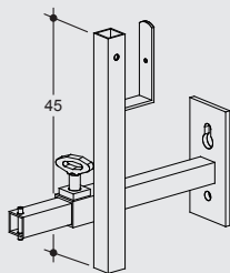
PROTECTO Pfostenhalter vari PROTECTO post holder vari
