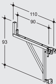
HT Laufkonsole Walkway bracket
