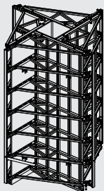
Säulenschalung 320/120 Column formwork 320/120
