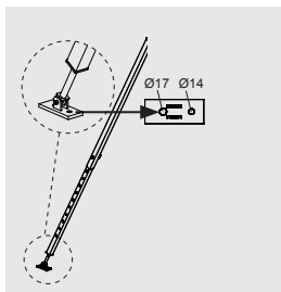
Richtstrebe P330 Aligning strut P330
