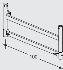
ID Ausgleichsrahmen 33 ID adjustment frame 33
