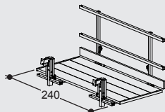
MANTO Betonierbühne MANTO pouring platform
