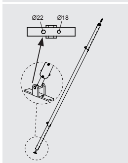
Richtstrebe Alu 10 Aligning strut Alu 10
